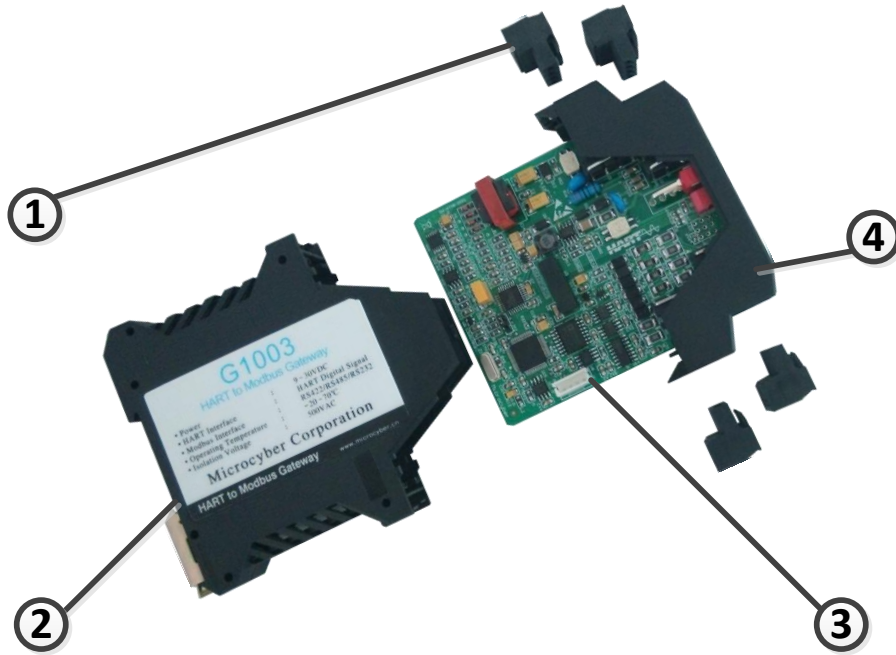
图 1.3 网关结构图
