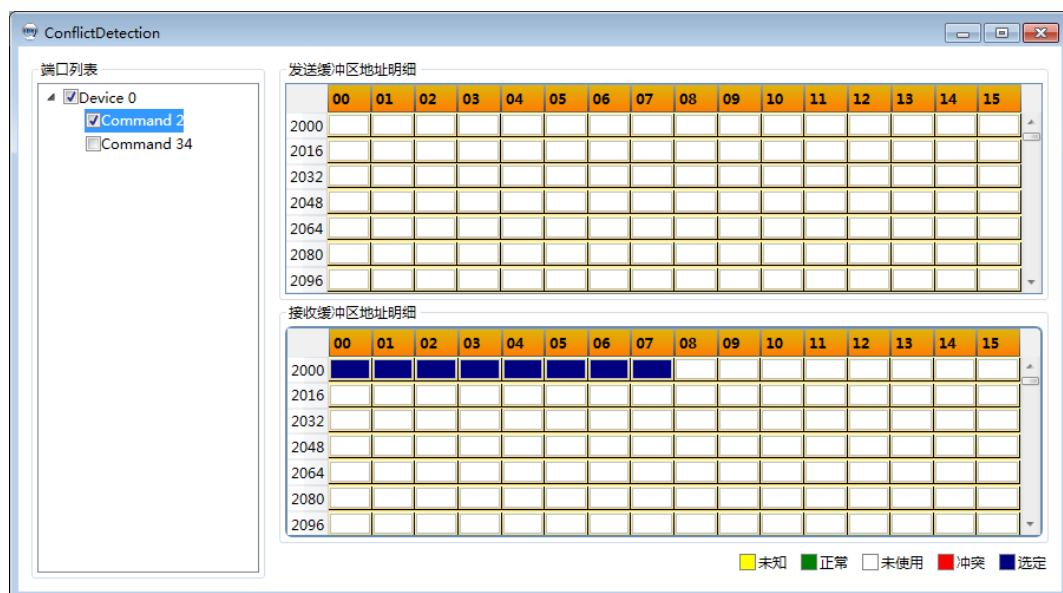
图 4.9 地址冲突检测界面
