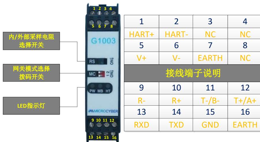
图 2.2 网关硬件接口图
