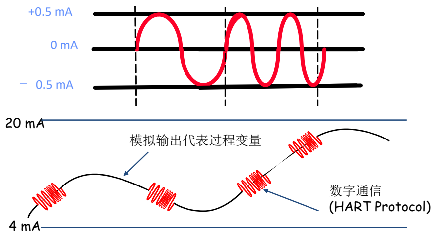
图 2.1 HART 物理层图示
