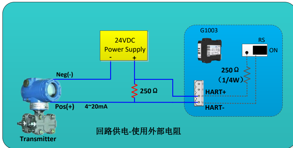
图 2.3 回路供电-使用外部电阻
