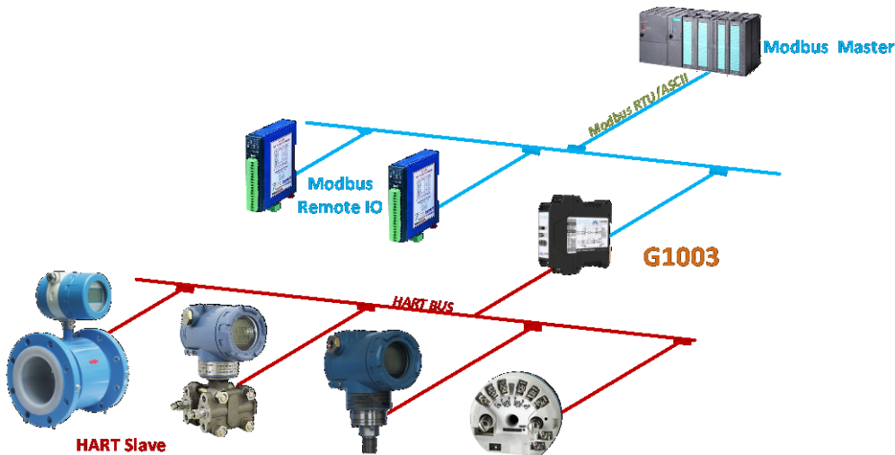
图 3.1 网关应用拓扑连接
