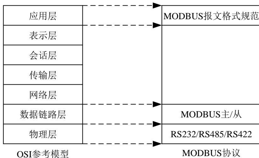
图 3.1 Modbus 协议模型
