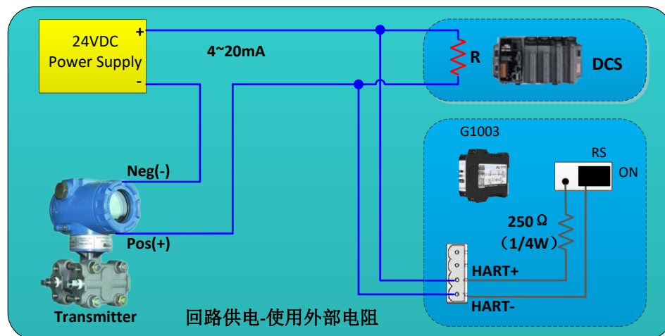
图 2.5 回路供电-使用外部电阻
