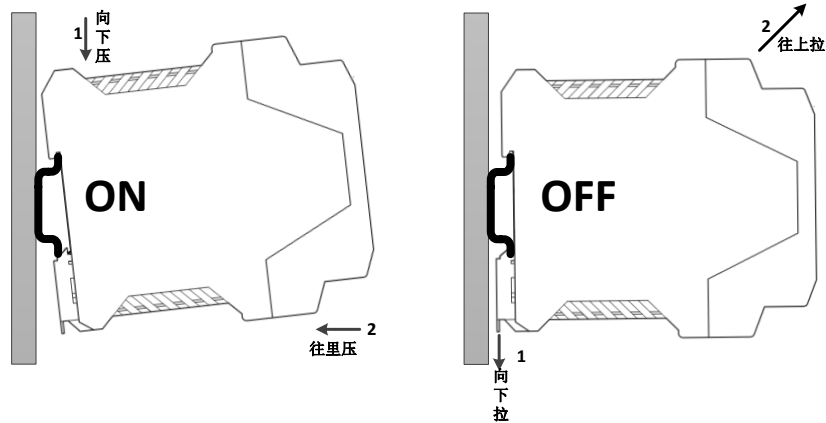
图 2.1 DIN 导轨安装图
