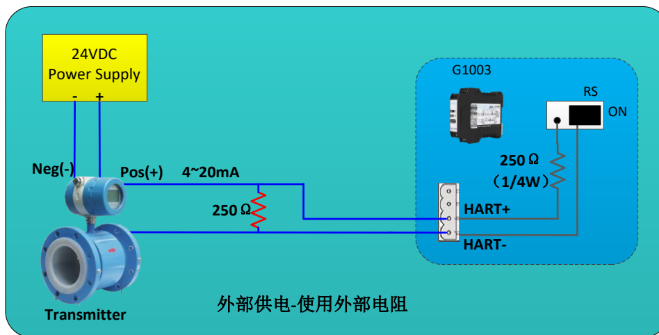
图 2.4 外部供电-使用外部电阻
