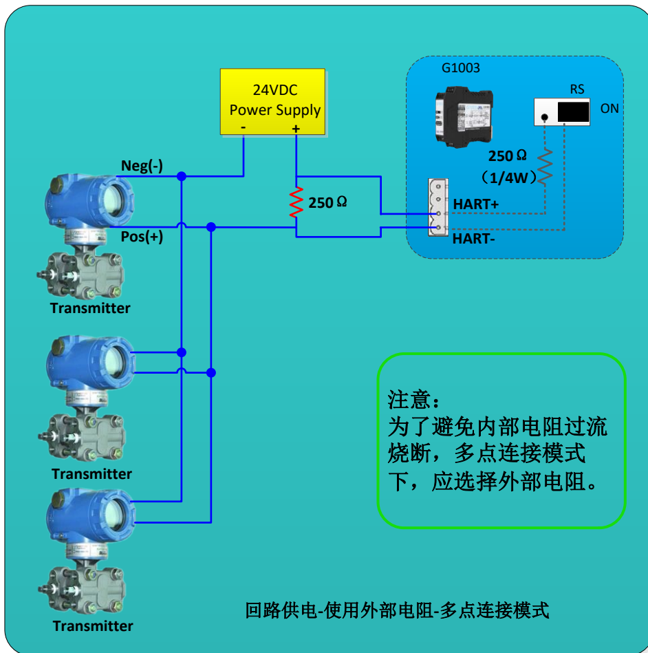
图 2.6 回路供电-使用外部电阻-多点连接模式
