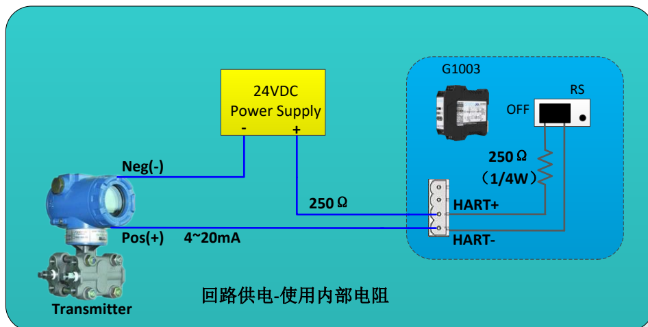
图 2.7 回路供电-使用内部电阻
