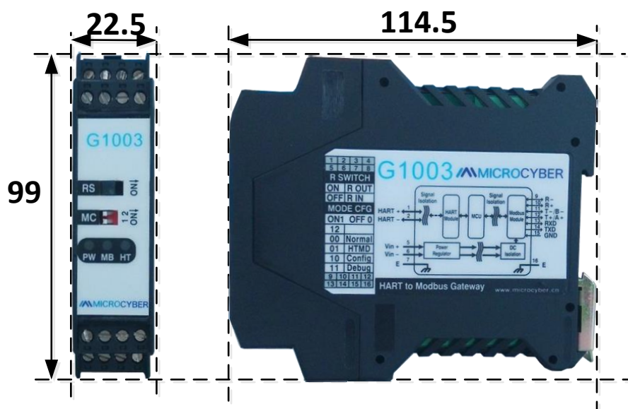
图 1.2 网关外形尺寸图 (114.5*99*22.5, 单位 mm)
