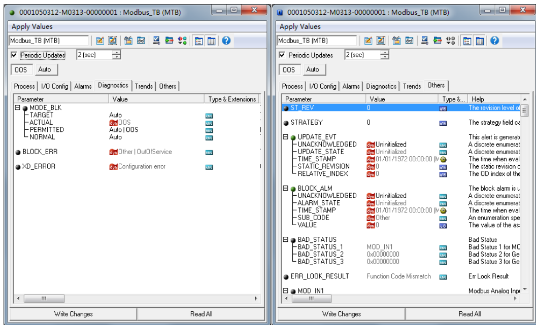
图 4.15 变换块 OOS 情况 3
