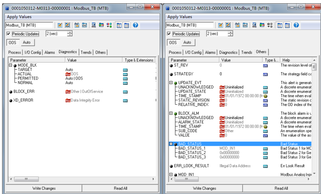
图 4.18 变换块 OOS 情况 6
