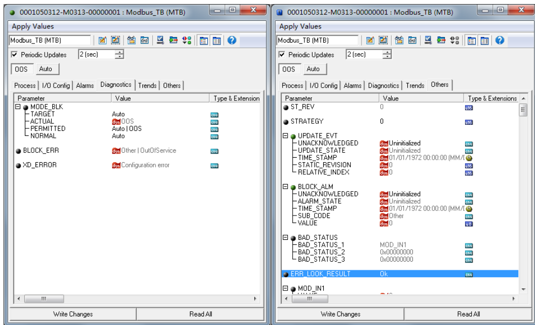
图 4.13 变换块 OOS 情况 1
