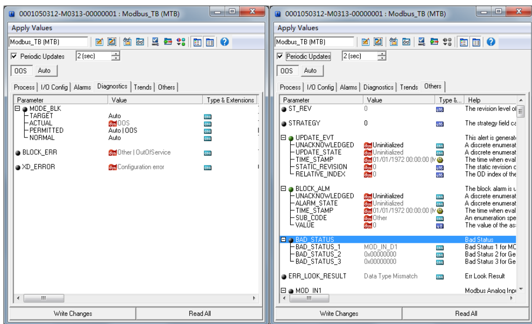
图 4.16 变换块 OOS 情况 4
