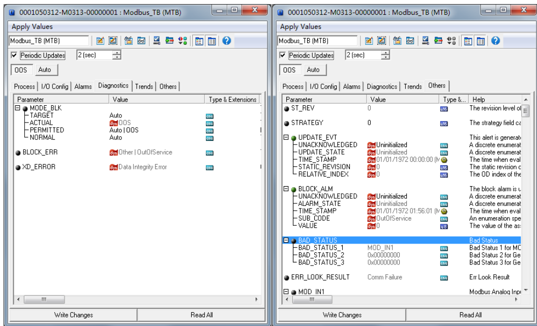
图 4.17 变换块 OOS 情况 5
